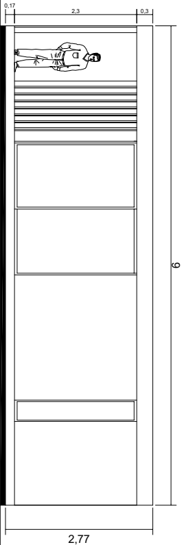
FACHADA NORTE
